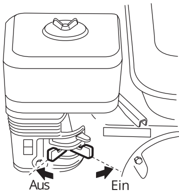
Kraftstoffhahn
