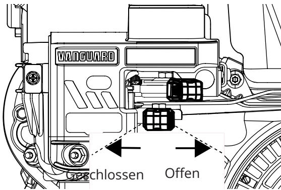
Kaltstarteinrichtung
