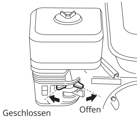
Kaltstarteinrichtung
